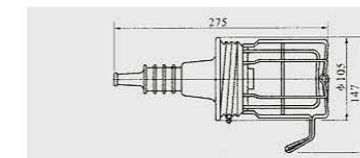
白熱手揚げ灯: WCSD2 / Incandescent portable light 製品サイズ: φ 105 × 275 製品特長: 下記
