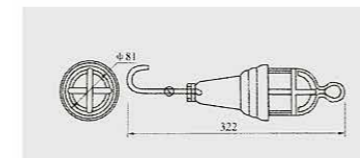
白熱作業灯: WCSD1 / Incandescent portable light 製品サイズ: φ 81 × 322 製品特長: 下記↓
