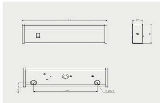
WJTL04-1・WJTL04-1C / LED bedside light 製品サイズ：331.5 × 90 × 40
