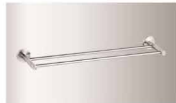
タオル掛け (2本) : WXP1102 / Double towel bar サイズ：556 × 124 × (φ49) 材質：SUS304 ステンレス 表面：鏡面仕上げ / ヘアライン仕上げ / Material: Stainless steel
