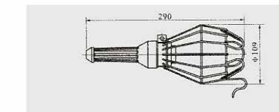
白熱手揚げ灯: WCSD3 / Incandescent portable light 製品サイズ: φ 102 × 290 製品特長: 下記↓
