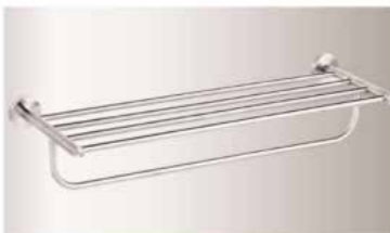
タオルラック : WXP1104 / Towel rack サイズ：610 × 214 材質：SUS304 ステンレス 表面：鏡面仕上げ / ヘアライン仕上げ / Material: Stainless steel
